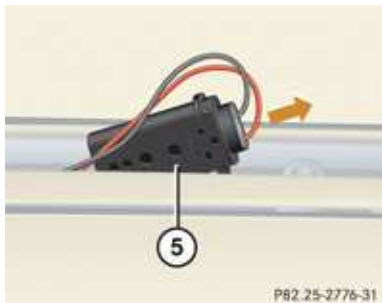
⑤ Anschlussstecker Dachzeichen
