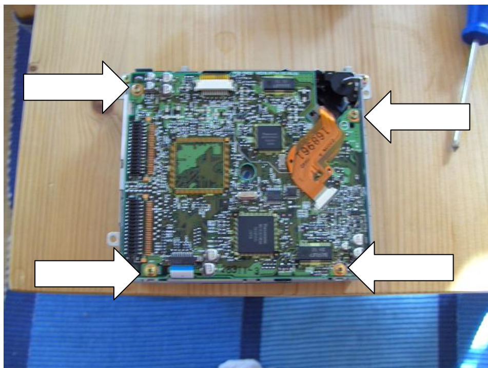
Ansicht Platinenseite
